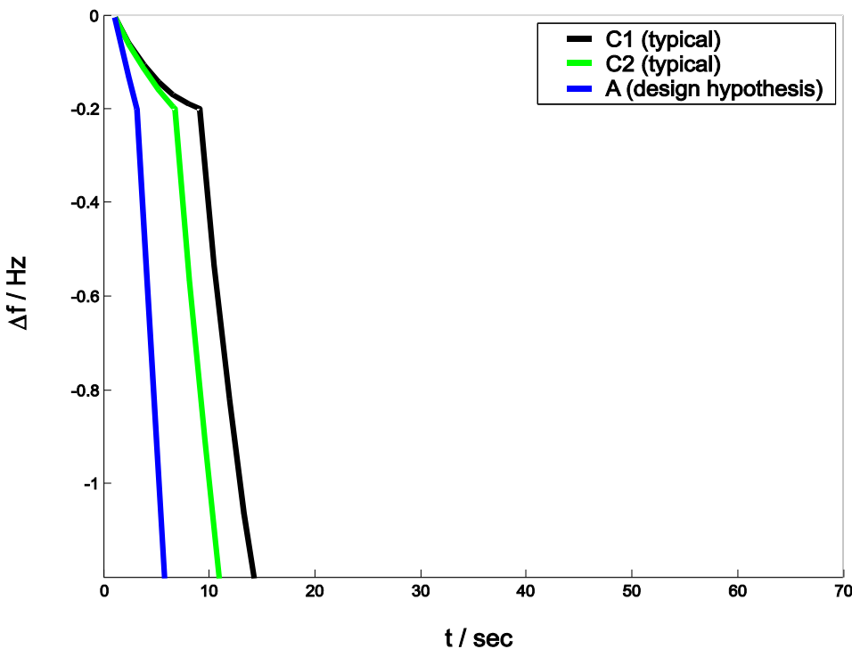
Abbildung 10: Frequenzverhalten des Netzes bei Bedingungen wie in den vorherigen Abbildungen, allerdings unter der Annahme, dass 10.000 MW dezentrale Leistung unterhalb von 49,8 Hz abschalten
