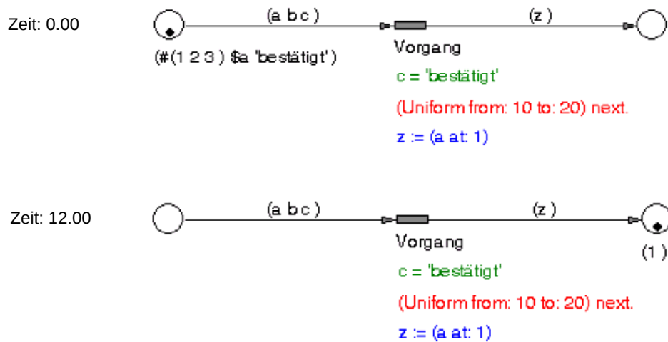
Abbildung 5.1: Beispiel für Inskriptionen einer Transition
