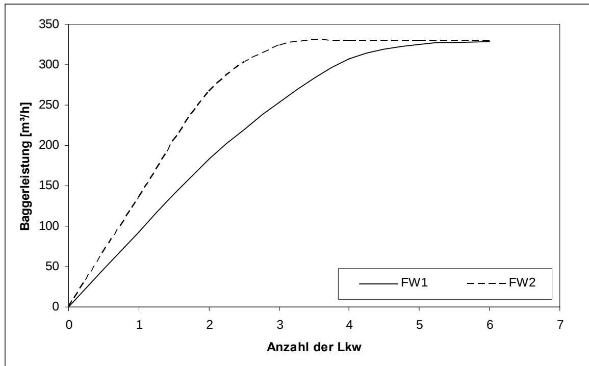
Abbildung 7.11: Leistung des Baggers CAT 345, in Abhängigkeit von der Anzahl der Lkw bei zwei alternativen Förderwegen
