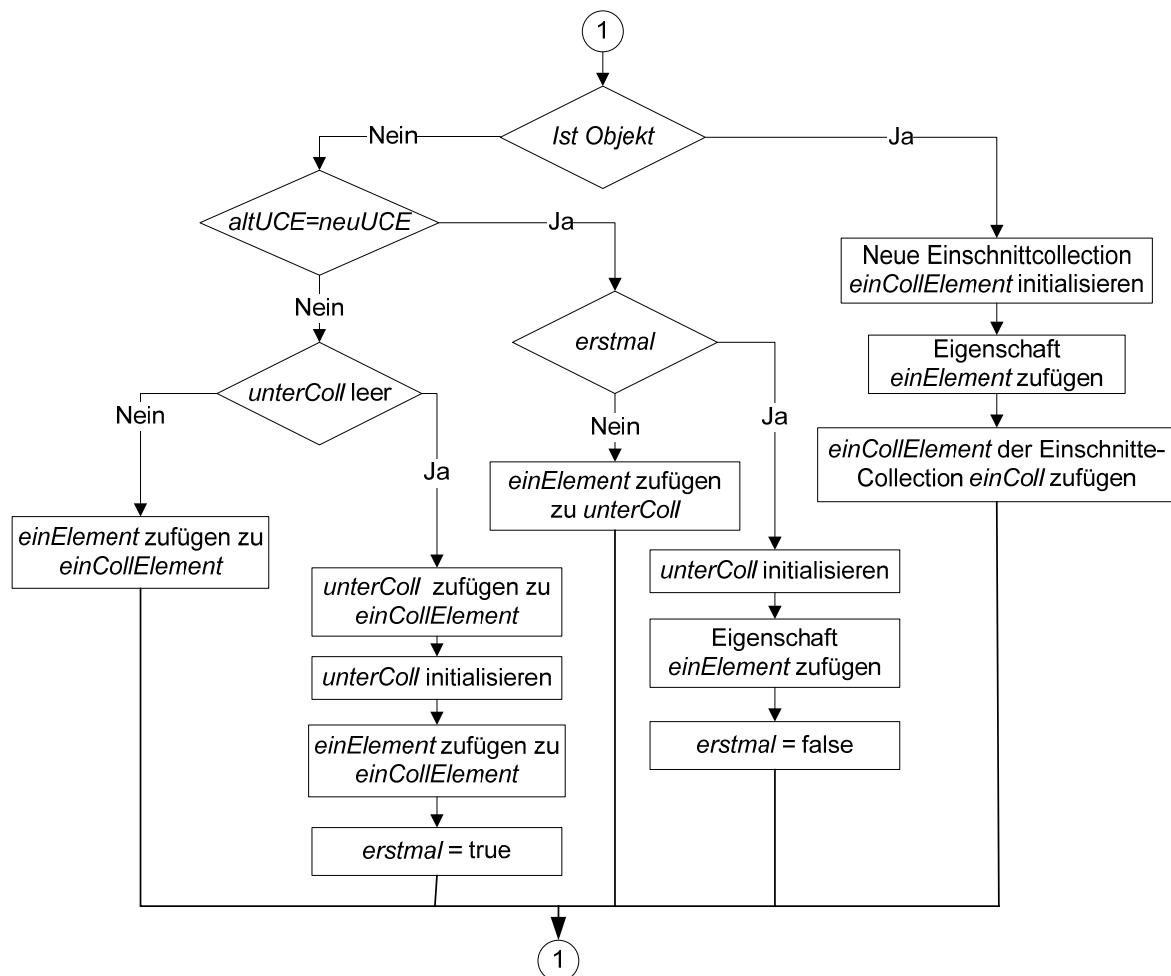
Abbildung 5.12: Datentransfer vom SRM zum Simulationssystem – XML-Elemente
