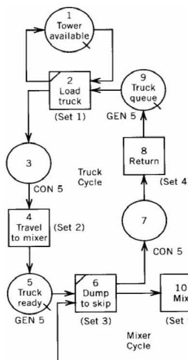
Abbildung 2.3: Ausschnitt aus einem CYCLONE Beispielsmodell und Netzkomponente ( Halpin und Woodhead 1998 S. 190 )
