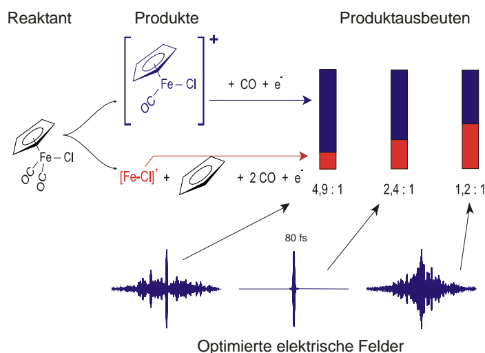
Bild 5.3: Adaptive Quantenkontrolle des [\text{CpFe}(\text{CO})\text{Cl}]^+ / [\text{FeCl}]^+ Produktverhältnisses. Im oberen Teil sind die relativen Produktausbeuten der in Betracht gezogenen Produktkanäle dargestellt. Im unteren Teil ist der Zeitverlauf der elektrischen Felder der Laserpulse dargestellt. Links ist das optimierte Feld für die Maximierung des Produktverhältnisses dargestellt, rechts das Feld für die Minimierung. Das Feld eines bandbreitebegrenzten 80 fs Laserpulses – das zu einem intermediären Produktverhältnis führt – ist zum Vergleich dargestellt.
