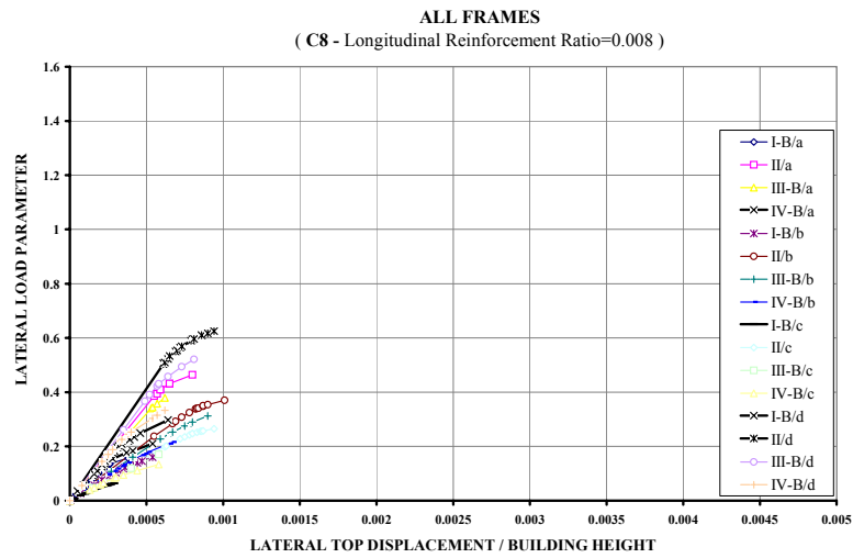
Figure 3.5.(d) The P-\delta/H curves
