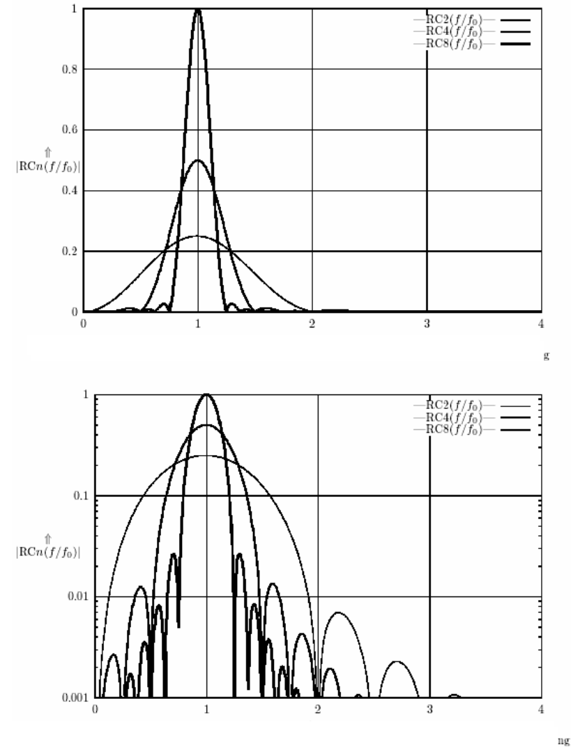
Time Spectrum of the RC2, RC4, and RC8 Excitation Function / Zeitspektrum des RC2-, RC4- und RC8-Anregungsimpulses
