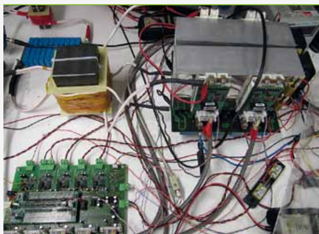
Laboraufbau der bidirektionalen DC-Stromversorgung Experimental setup of the bidirectional DC power supply
