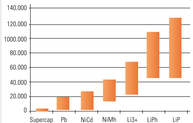
Selbst-Hubhöhe [m]
