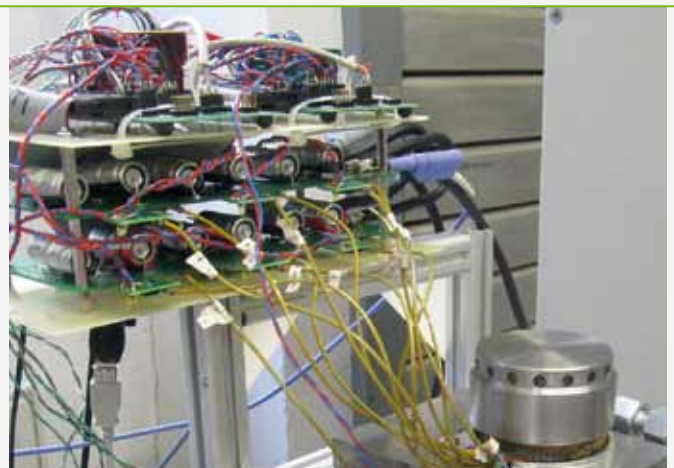
Laboraufbau des Hilfsantriebssystems Experimental setup of the auxiliary drive system
