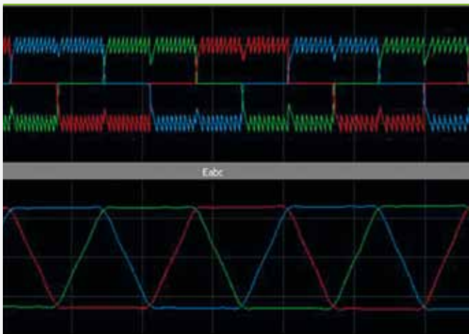
Strom-, Spannungsverläufe einer dreiphasigen BLDC-Maschine Current- and voltage-profiles of a three phase BLDC-Machine
