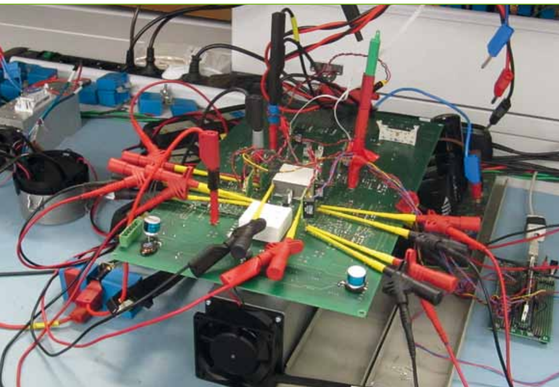
Laboraufbau eines DC-DC Wandlers Experimental setup of one DC-DC converter
