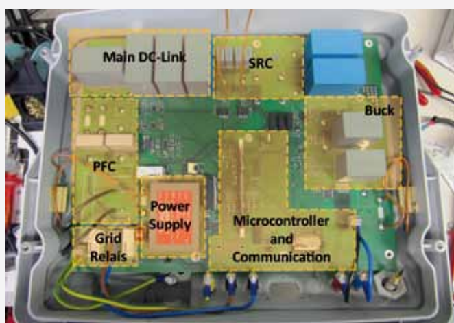
Hauptplatine des Ladegeräts Main circuit board of the charger
