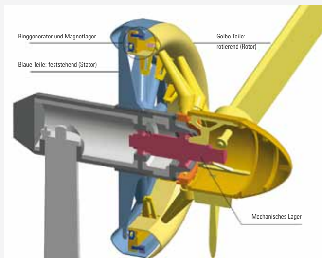
Schnittbild des neuen WEA-Konzepts Sectional view of the new WEC-concept
