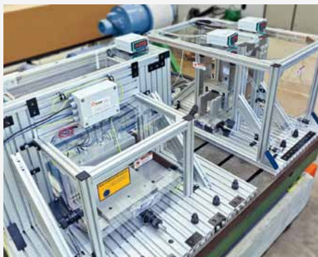
Versuchsmodelle zur Messung von Normal- und Magnetlagerkräften Test models for the measurement of normal and magnetic bearing forces
