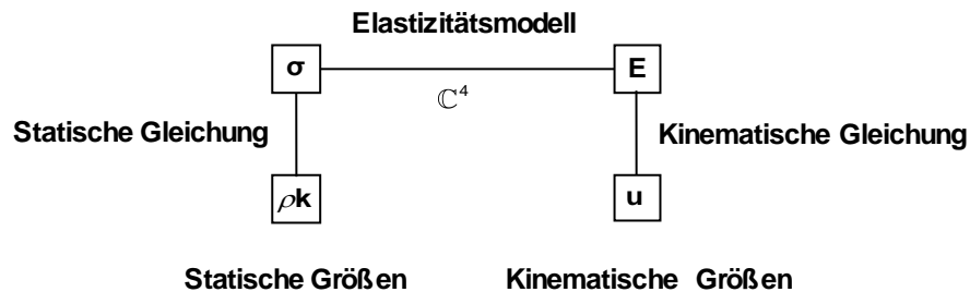
Abb. 3.1.-1: Tonti-Diagramm
