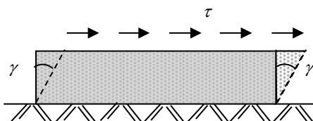
Abb. 3.2.-1: Einfache Schubbelastung
