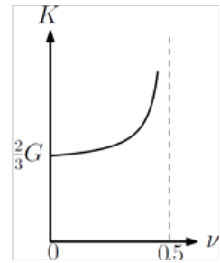
Abb. 3.2-4 : Verlauf K über \nu
