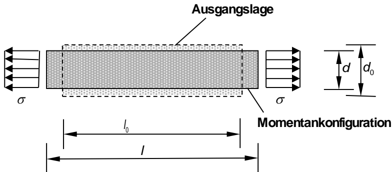
Abb. 3.2.-2: Einachsige Zugbelastung
